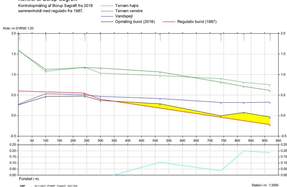
Figur 1. Længdeprofil for Borup Søgrøft med regulativ- og opmålingsdata
